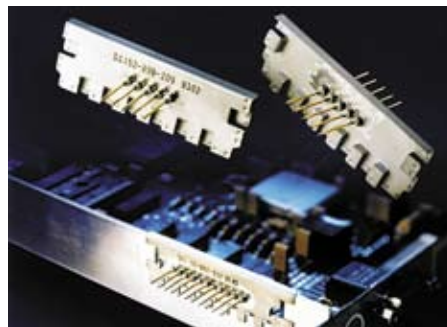
Рис. 6. Типовой пример монтажа сборки серии Easy Mate Filter Plates
