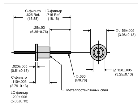
Рис. 9. Чертеж корпуса серий SCI-9900 и SCI-9980
